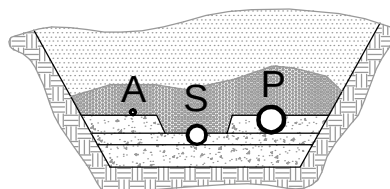
COUPE 1-1
